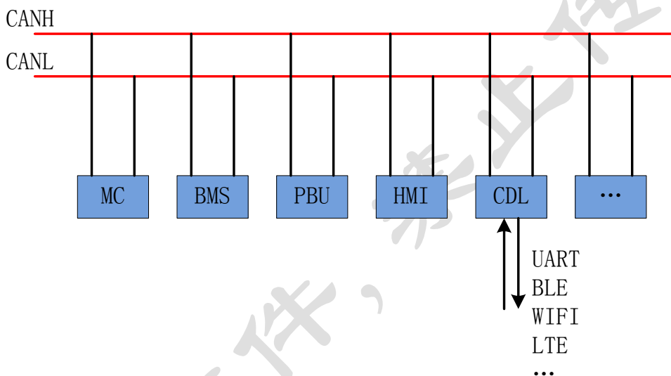
图1 系统通信接口示意图
