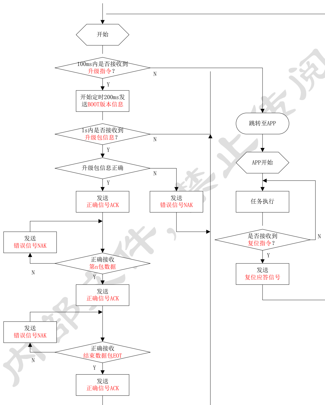
图2 升级流程图
