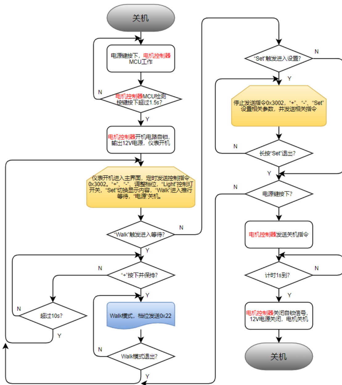
图7 系统架构 2 仪表工作流程图
