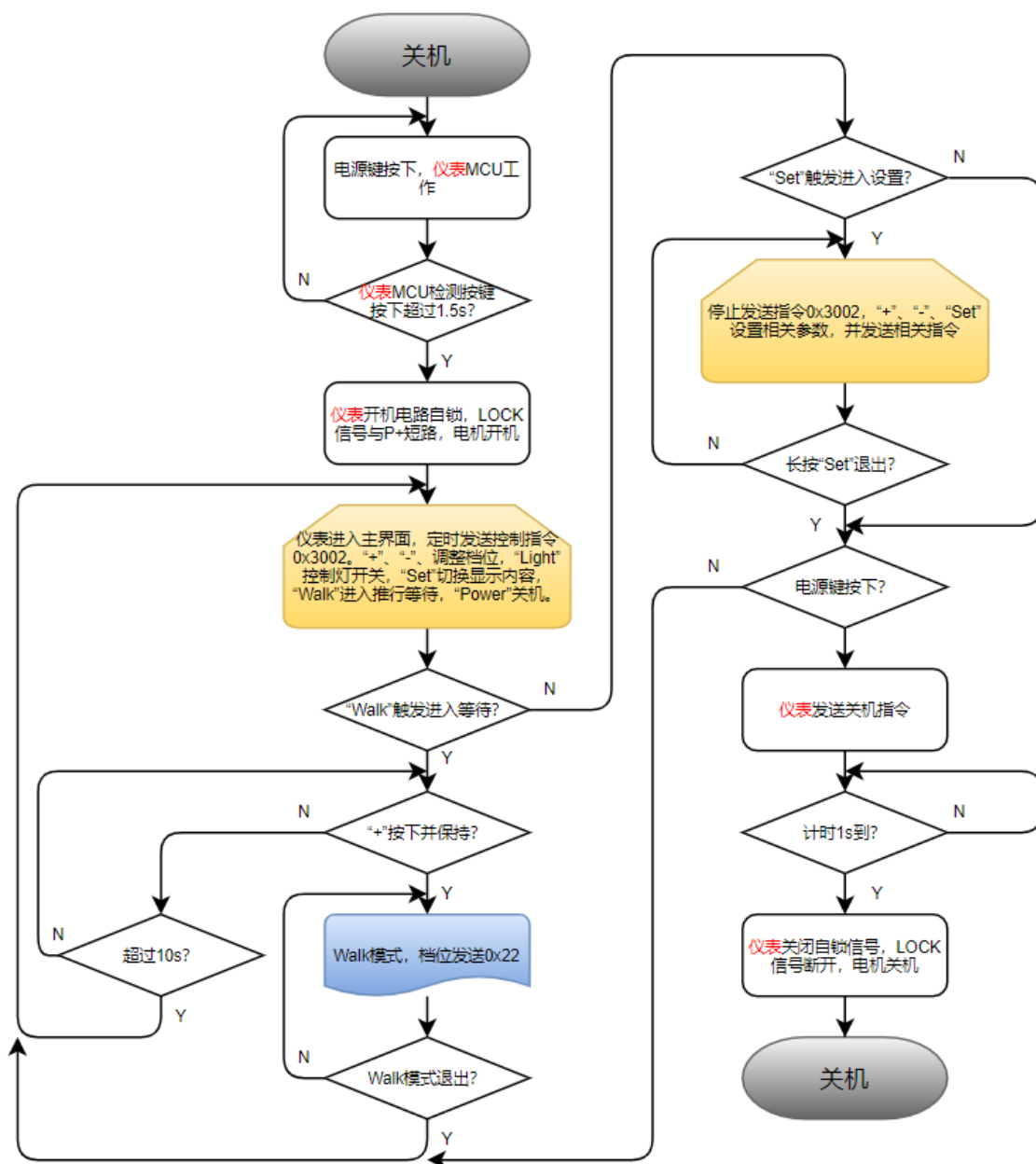
图6 系统架构 1 仪表工作流程图
