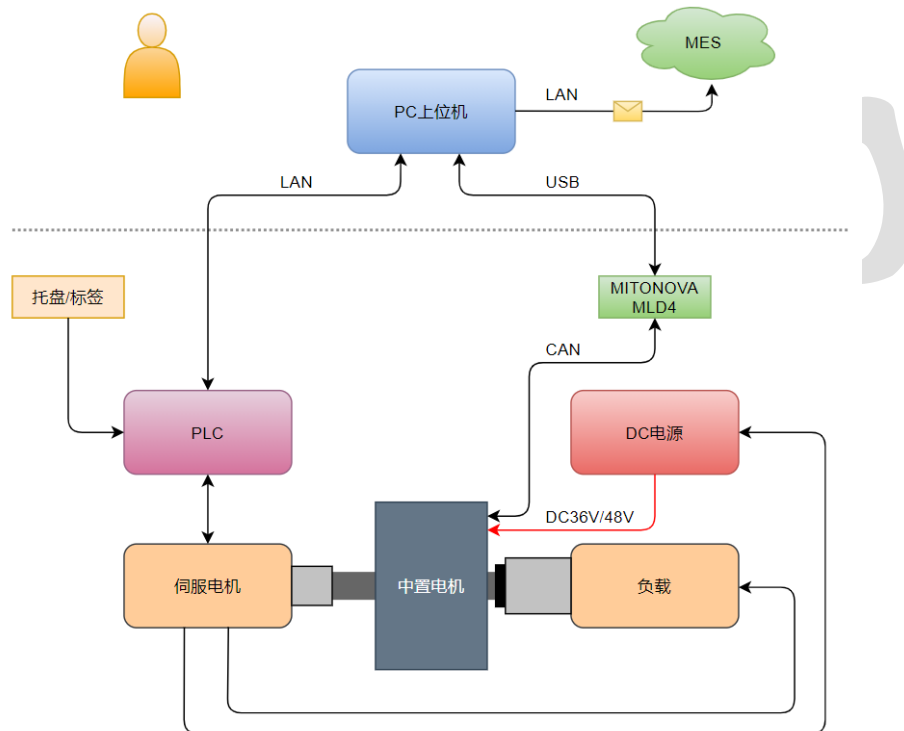
图1 标定设备组成示意图
