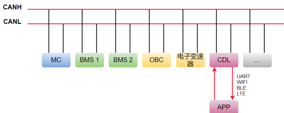
图1 系统通信接口示意图
